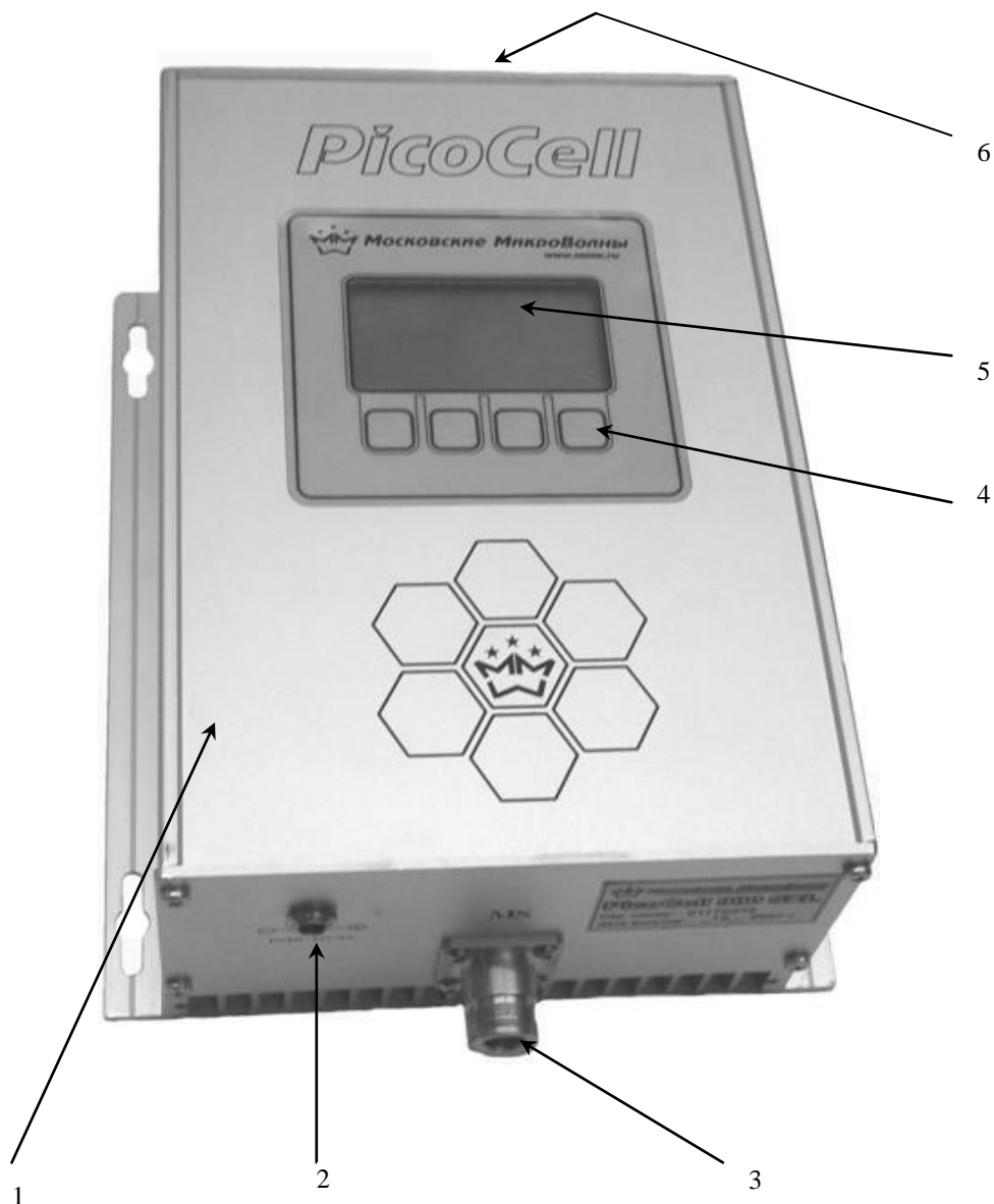
Рис.1 Ретранслятор PicoCell 1800 SXL
